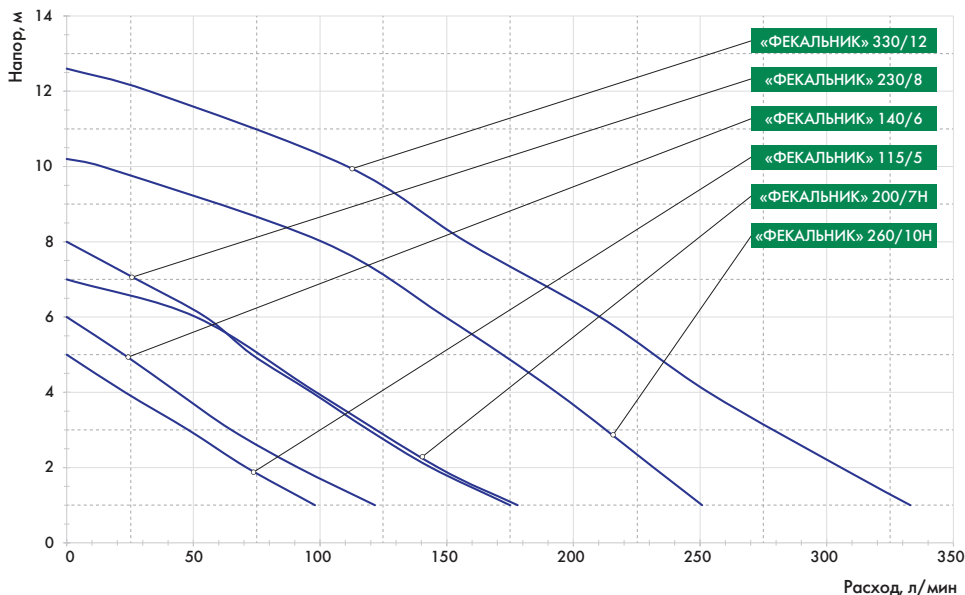
Графики расходно - напорных характеристик насосов серии «ФЕКАЛЬНИК»*
